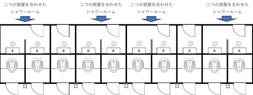
ベトナム中部、Quang Nam省、Tay Giang郡、A Dau小中学校シャワールーム・トイレ改修工事
